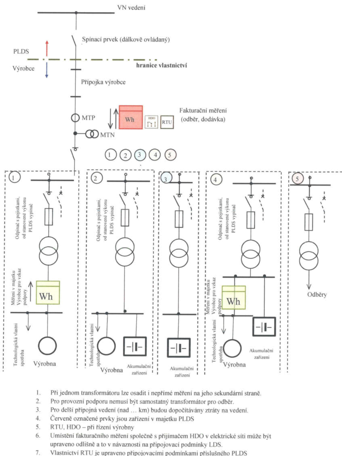
Obr.12 Připojení výroby elektřiny a akumulárního zařízení z nadzemního vedení vn přípojkou výrobce
