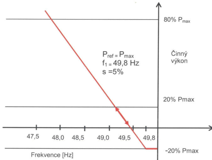
Obr.7 Frekvenční odezva činného výkonu na podfrekvenci u akumulárního zařízení.
